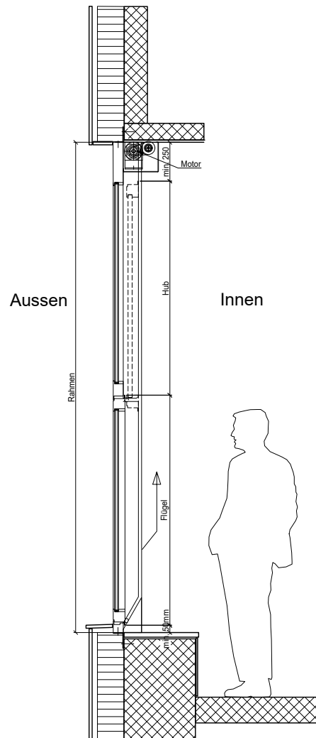
Vertikalschnitt
