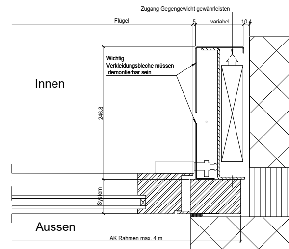
Horizontalschnitt
